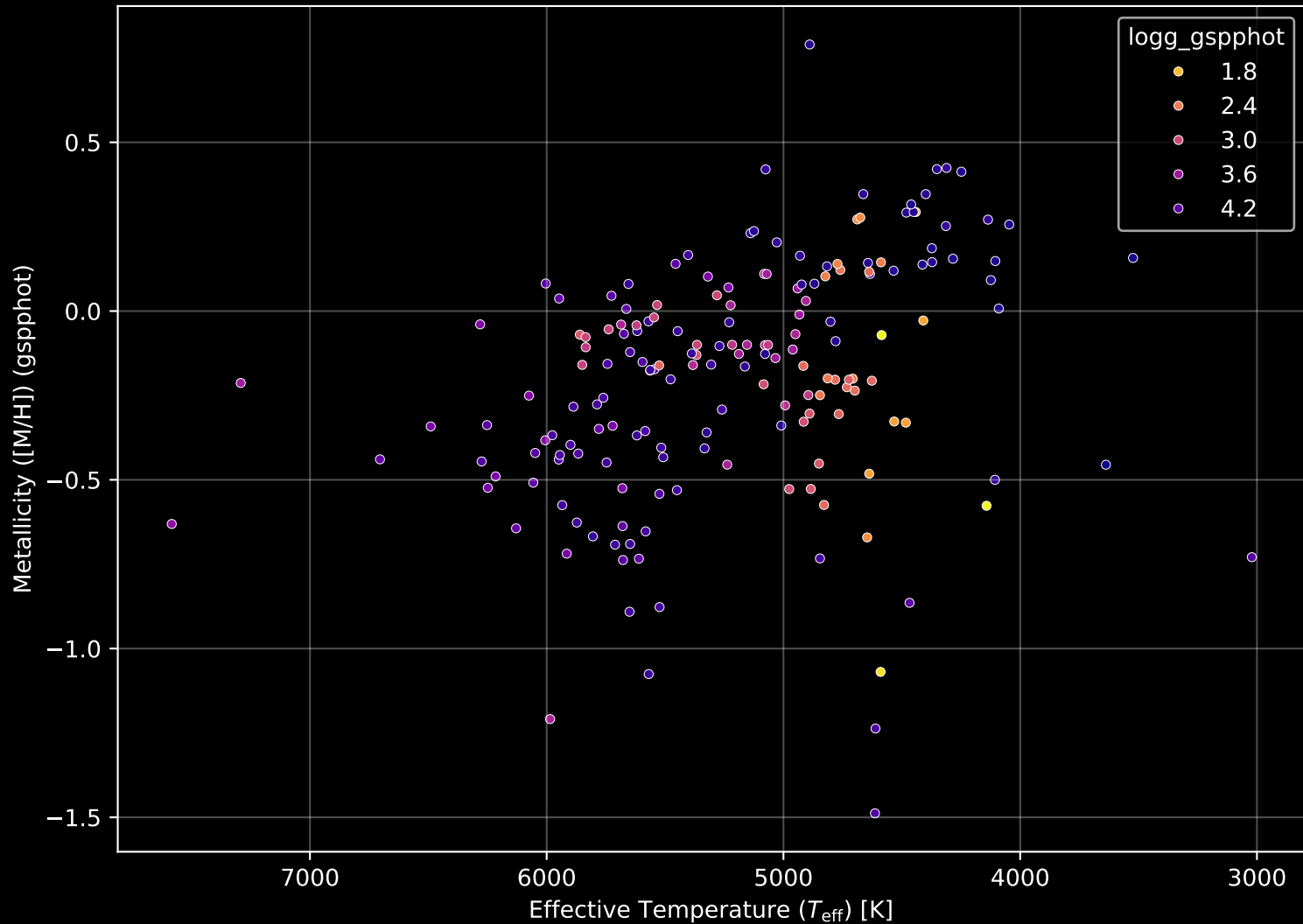
APOGEE DR17 Field: [323+60_MGA] Stellar Population Parameters (n= 180)
